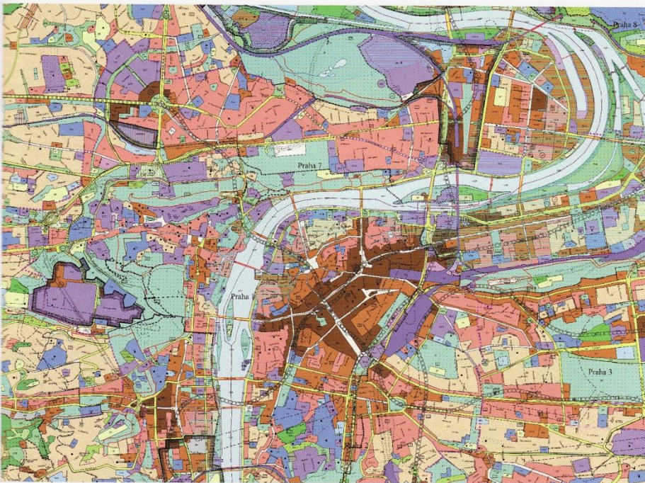
Detail – výkres č. 4 územního plánu Prahy, plochy v celoměstském systému zeleně jsou vyjádřeny tečkovanou šrafou
